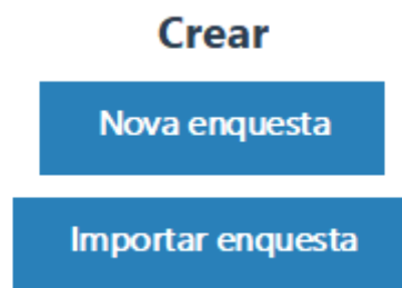
Figura 12. Botons creadors
